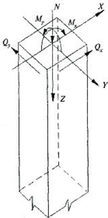
Рисунок 8.1 - Схема усилий, действующих на выделенный стержневой элемент
